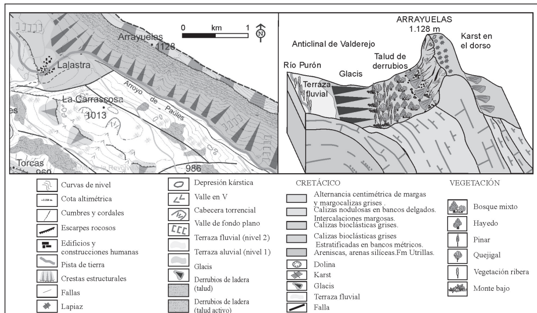
Figura N° 5 Mapa geomorfológico del lugar de interés geomorfológico n° 2. Arrayuelas
